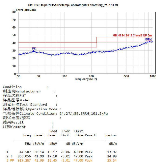
图 5-7 辐射测试垂直方向
