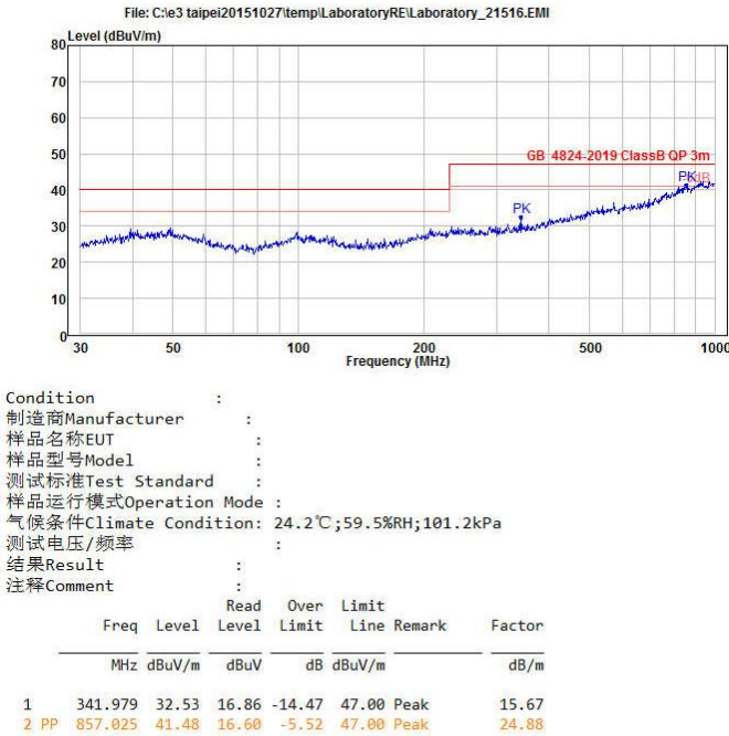
图 5-6 辐射测试水平方向
